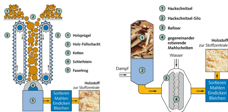
Abbildung 7-6: Mechanische Holzstoffherstellung (links) und thermochemische Holzstoffherstellung (rechts)
