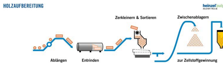
Abbildung 7-4: Holzaufbereitung
