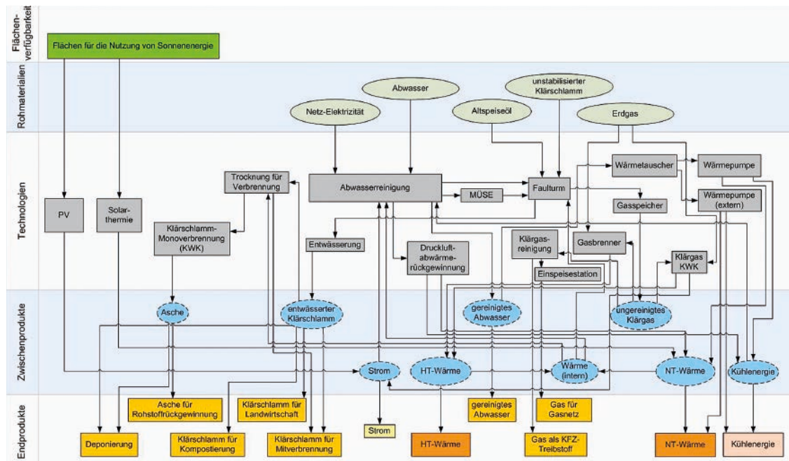
Abb. 30: Maximales Technologienetzwerk zur Optimierung einer Kläranlage (adaptiert nach Kindermann und Kollmann, 2015).
