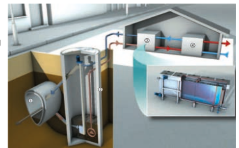
Abb. 10: System zur Wärmeabgewinnung von Kanalabwasser außerhalb der Kanalleitung; Systemdarstellung Huber ThermWin. HUBER SE.
