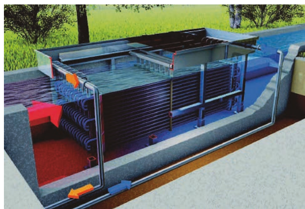
Abb. 14: Wärmetauscher im Ablaufkanal. HUBER SE, Berching.
