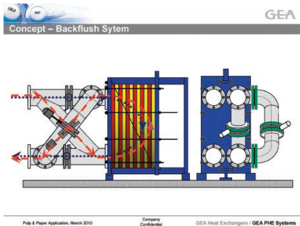
Abb. 12: Backflush (Rückspüleinrichtung). Kelvion Holding GmbH, Bochum.
