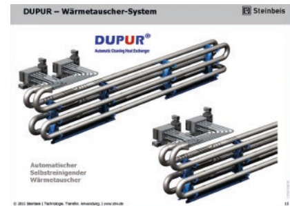
Abb. 11: Systemdarstellung selbstreinigender Wärmetauscher für den Einsatz vor der Kläranlage. Jaske & Wolf Verfahrenstechnik GmbH.
