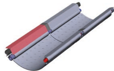
Abb. 9: Moderne Wärmetauscher (Therm liner Form B Prinzipdarstellung) können auf die Sohle eines bestehenden Kanals montiert werden und dem Abwasser Wärme entziehen. Uhrig Kanaltechnik GmbH.
