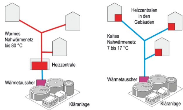
Abb. 15: Prinzipschema Warmes Netz / Kaltes Netz. Eigene Bearbeitung nach Müller et al. 2005, Tracey Saxby, IAN Image Library.
