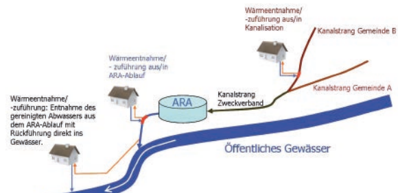
Abb. 2: Schematische Darstellung von Wärmeentnahmen und -einträgen. (Koch et al. 2010). AWEL (Kanton Zürich).
